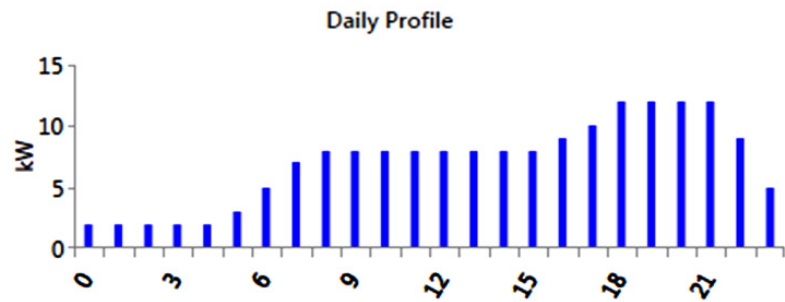
Fig. 10. Perfil diario de demanda comunitaria.
