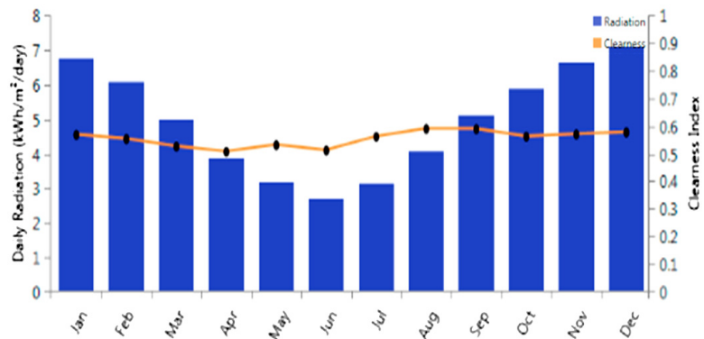
Fig. 11. Perfil de radiación solar mensual.
