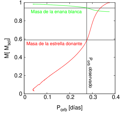
Figura 2: Cambio de las masas de ambas estrellas del sistema en función del período orbital.
