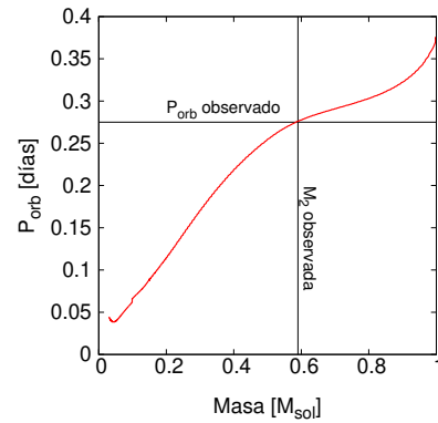
Figura 3: Evolución del período orbital en función de la masa de la estrella donante.
