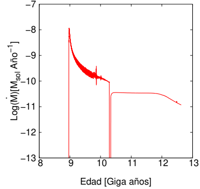
Figura 5: Tasa de transferencia de masa en función del tiempo.
