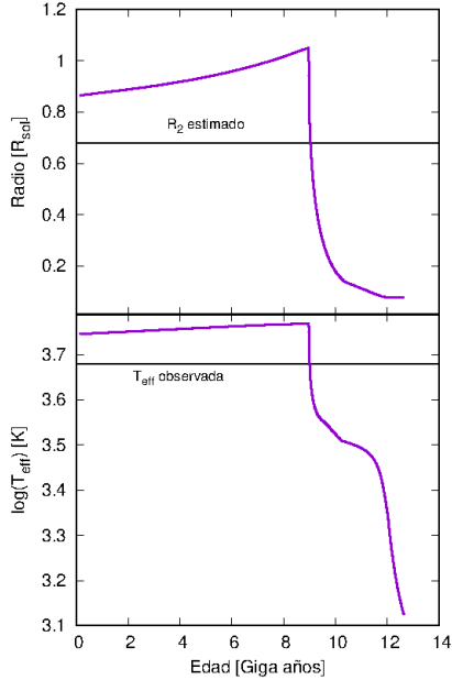
Figura 4: Evolución del radio ( panel superior ) y de la temperatura efectiva ( panel inferior ) de la estrella donante en función del tiempo.
