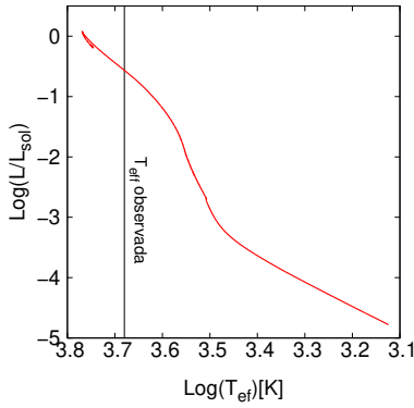
Figura 1: Diagrama de Hertzsprung-Russell para la estrella donante. La línea vertical indica el valor de la temperatura efectiva de la estrella donante en SS Cyg.
