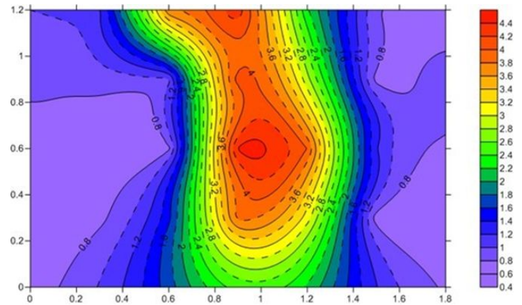
Figura 8: Perfil de velocidad a la salida de difusor y entrada de la cámara de secado.
