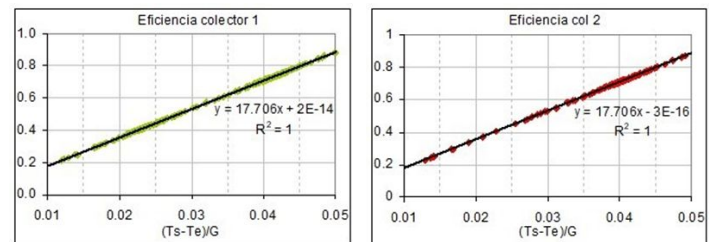
Figura 9: Cálculo de eficiencia de colectores ensayados, considerando (T_s - T_{amb})/G
