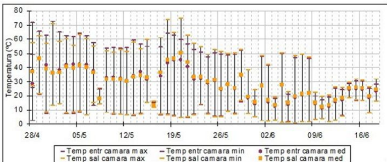
Figura 5: Temperatura de flujo en la entrada y salida de la cámara de secado.
