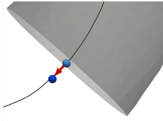
Figura 4: Ejemplo de puntos de corte sobre la línea central (en negro) seleccionados automáticamente por el algoritmo. Sobre ellos se crean los planos perpendiculares a la superficie para efectuar el aislamiento. La flecha roja indica la dirección seguida para fijar el segundo punto de corte.
