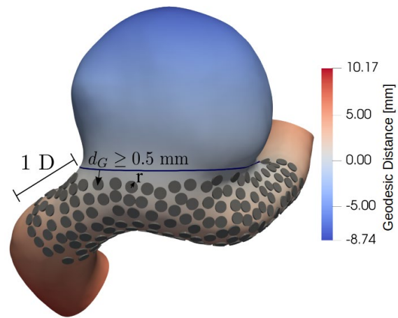
Figura 7: Detalle de los puntos de carga. Cada uno de ellos tiene un radio r de 0.25 mm (para visualización). Los puntos de carga están limitados a una región cercana al cuello (“chaleco”), definida con un algoritmo similar al de corte a una distancia de 1 D ( D = diámetro interno).
