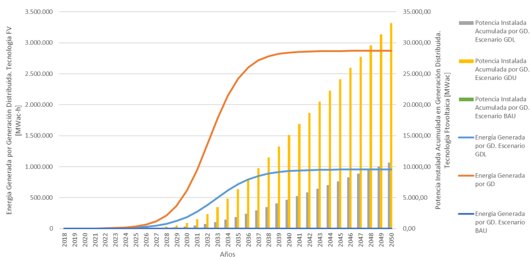
Figura 2: Oferta de energía eléctrica por penetración de instalaciones de generación distribuida con tecnología fotovoltaica con conexión a la red, escenarios GDL y GDU (gráfico de líneas, eje izquierdo) y su potencia instalada acumulada (gráficos de barras, eje derecho). Elaboración propia.
