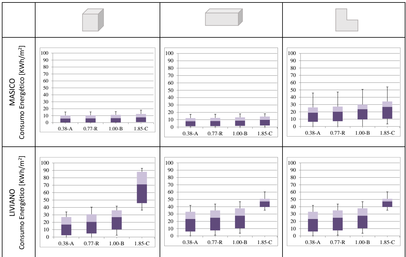
Figura 7. Consumos energéticos de enfriamiento de acuerdo a las modificaciones de U Techos , para Zona II Cálido –Chemical, La Rioja- Fuente: elaboración propia.
