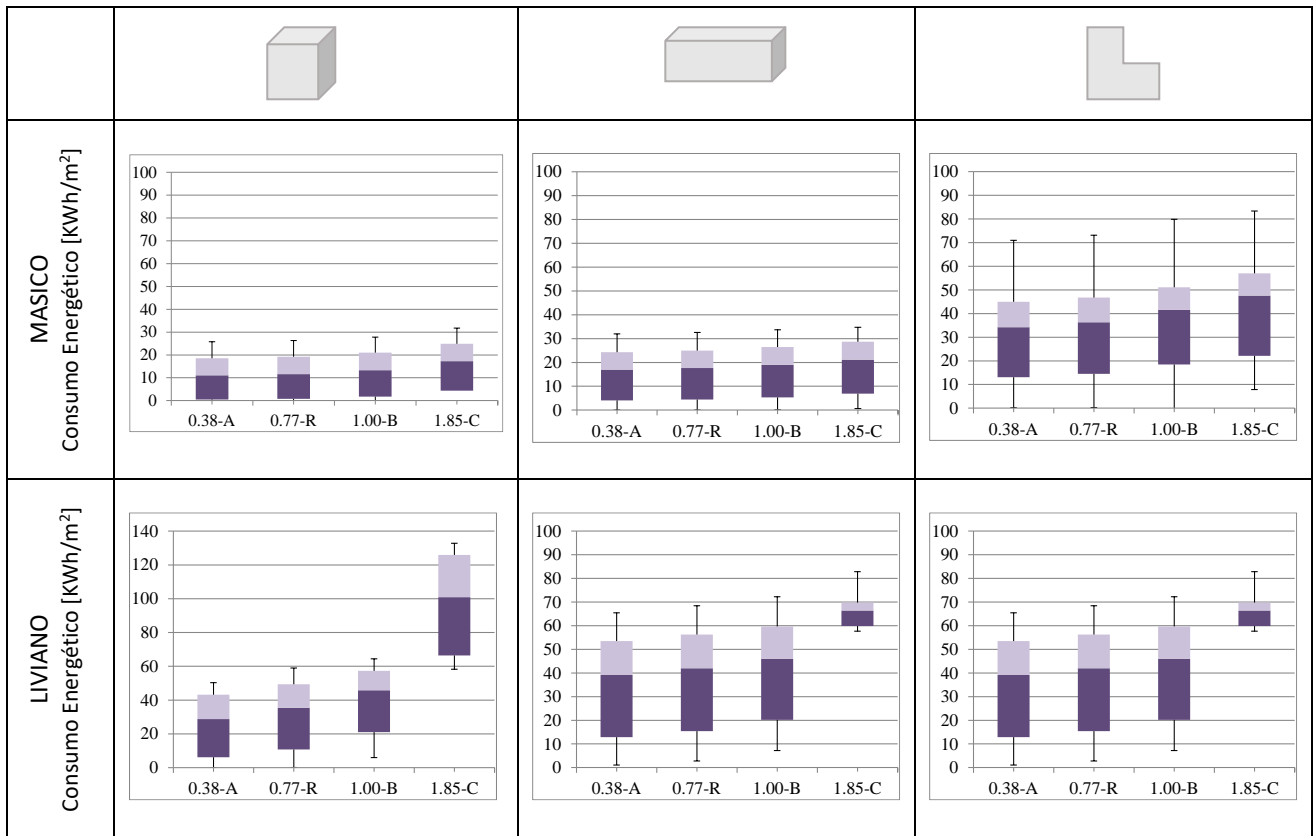
Figura 6. Consumos energéticos de enfriamiento de acuerdo a las modificaciones de U Techos , para Zona I Muy cálido –Formosa ciudad- Fuente: elaboración propia.
