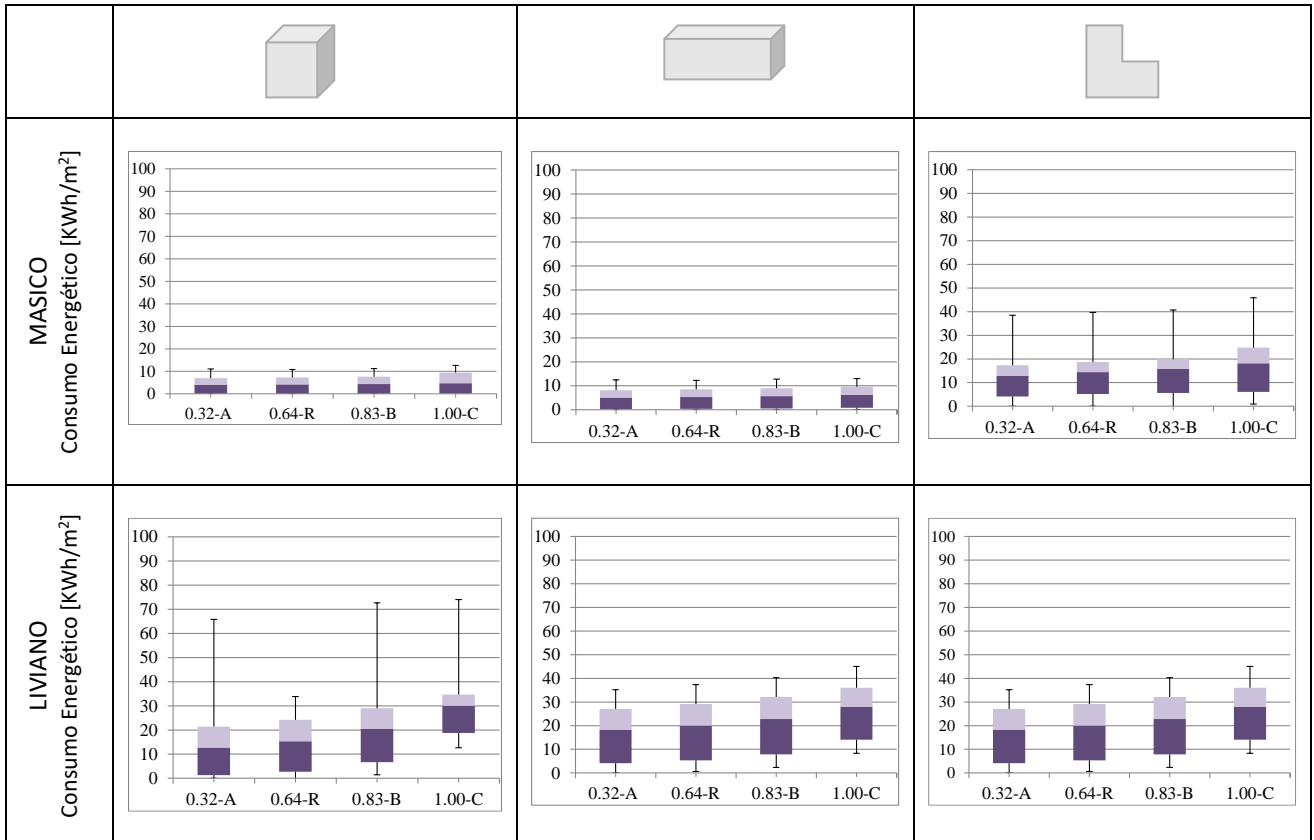
Figura 9. Consumos energéticos de enfriamiento de acuerdo a las modificaciones de U Techos , para Zona IV Templado frío – Mendoza, ciudad- Fuente: elaboración propia.
