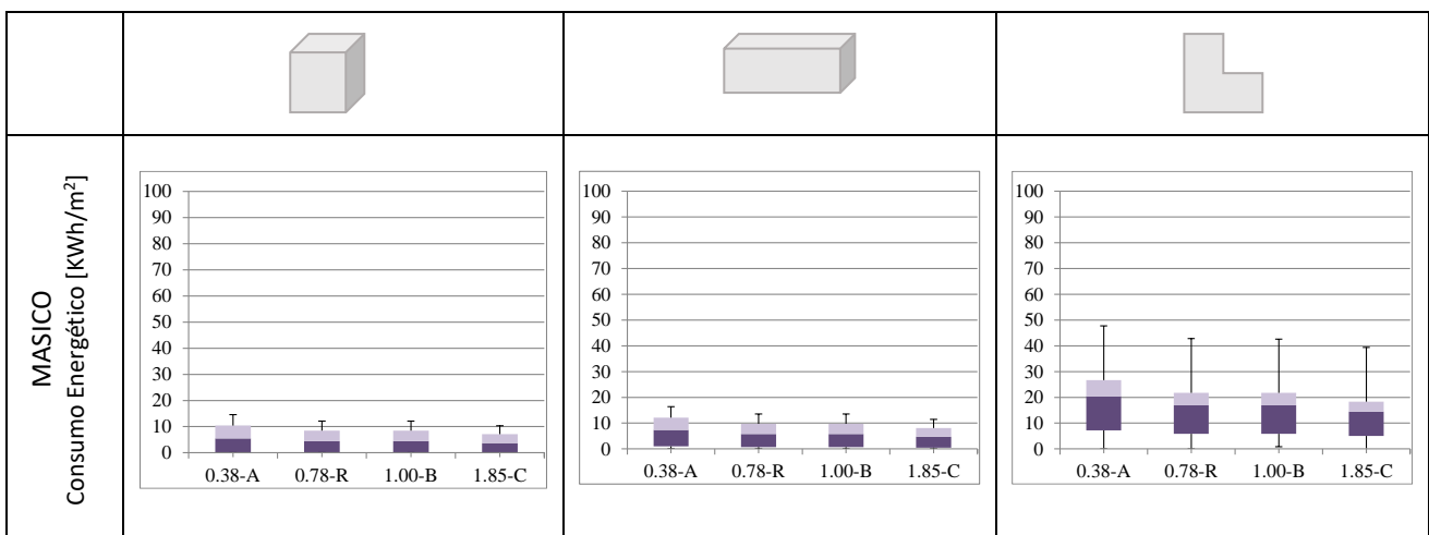
Figura 4. Consumos energéticos de enfriamiento de acuerdo a las modificaciones de U Muros, para Zona III Templado cálido –9 de julio, Buenos Aires- Fuente: elaboración propia.
