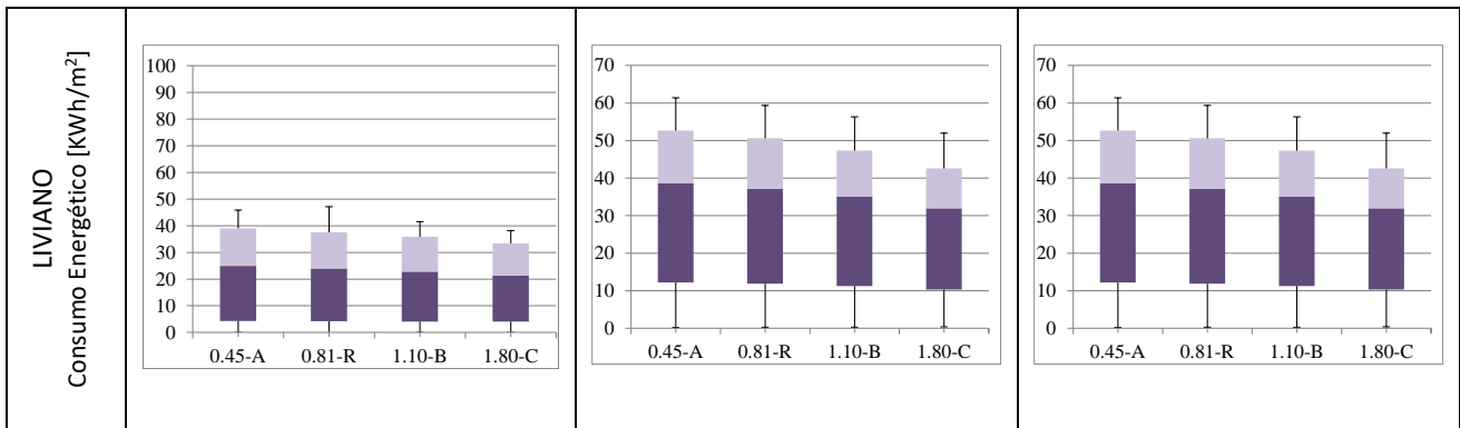
Figura 3. Consumos energéticos de enfriamiento de acuerdo a las modificaciones de U Muros, para Zona II Cálido –Chemical, La Rioja- Fuente: elaboración propia.
