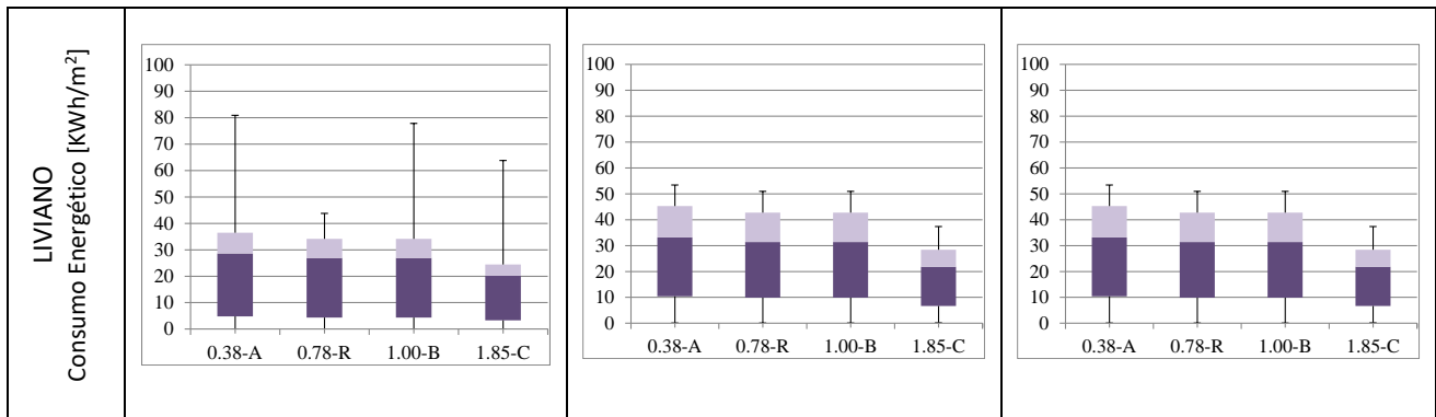
Figura 5. Consumos energéticos de enfriamiento de acuerdo a las modificaciones de U Muros, para Zona IV Templado frío – Mendoza, ciudad- Fuente: elaboración propia.
