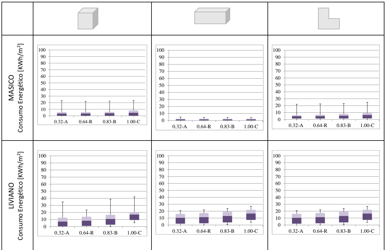
Figura 8. Consumos energéticos de enfriamiento de acuerdo a las modificaciones de U Techos , para Zona III Templado cálido –9 de julio, Buenos Aires- Fuente: elaboración propia.
