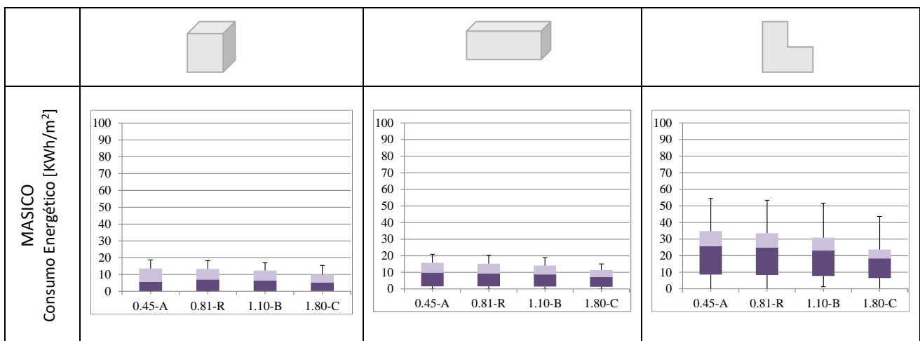
Figura 2. Consumos energéticos de enfriamiento de acuerdo a las modificaciones de U Muros, para Zona I Muy cálido –Formosa ciudad- Fuente: elaboración propia.
