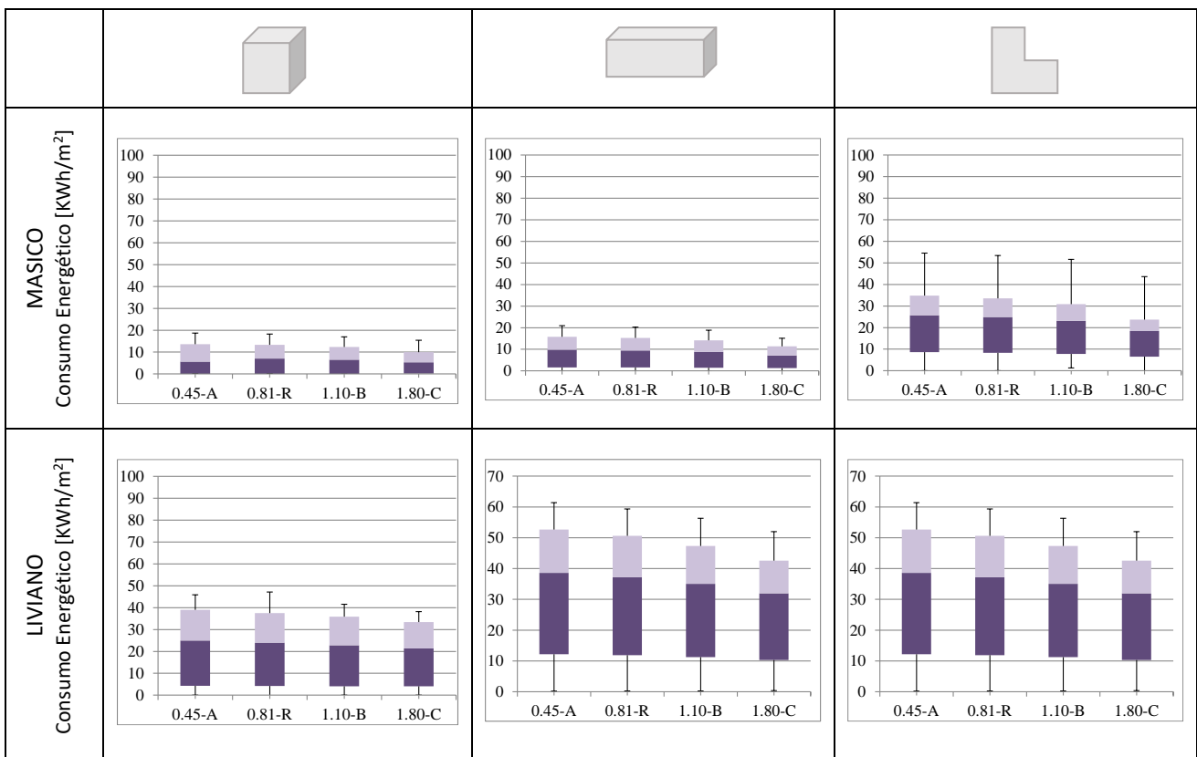
Figura 4. Consumos energéticos de enfriamiento de acuerdo a las modificaciones de U Muros, para Zona III Templado cálido –9 de julio, Buenos Aires- Fuente: elaboración propia.
