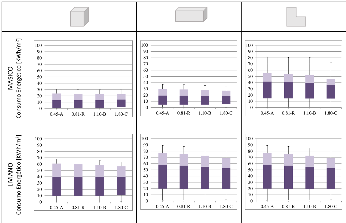
Figura 2. Consumos energéticos de enfriamiento de acuerdo a las modificaciones de U Muros, para Zona I Muy cálido –Formosa ciudad- Fuente: elaboración propia.
