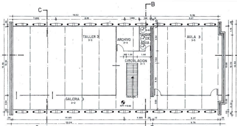
Fig. 8 Planta liberada y modulación respecto del orden estructural
