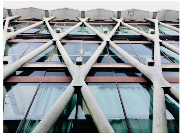
Fig. 5 Fachada Sur. Remate coronamiento losas plegadas
