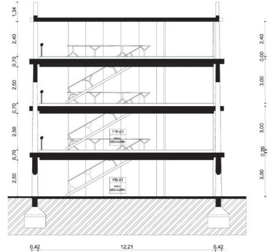
Fig. 9 Corte transversal con sistema de escaleras galería y salas.
