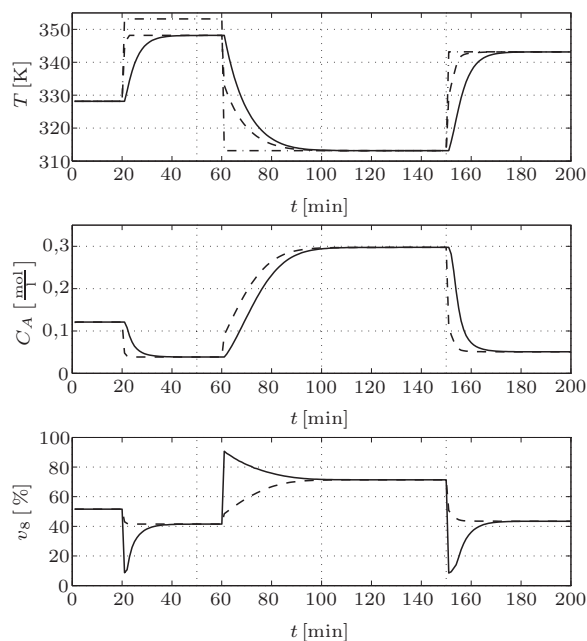
Figura 6: Ensayo de simulación de seguimiento de referencia con N = 6 . Arriba: temperatura (línea continua), referencia (línea de puntos y trazos) y referencia artificial (línea de trazos); centro: concentración (línea continua) y concentración artificial (línea de trazos); abajo: entrada (línea continua) y entrada artificial (línea de trazos).
