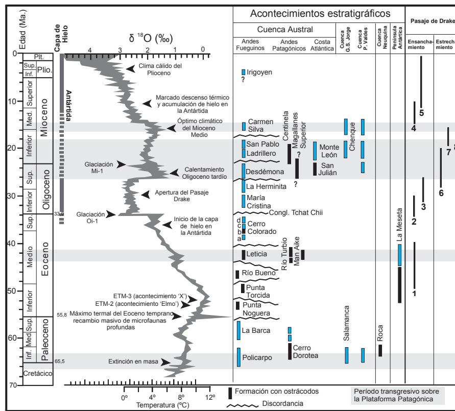
FIG. 2. Principales acontecimientos climáticos, tectónicos y estratigráficos que afectaron al sur de América del Sur durante el Cenozoico cotejados con la curva de \delta^{18}\text{O} de foraminíferos bentónicos de Zachos et al. (2001). Modificado de Zachos et al. (2001) y Lagabriele et al. (2009). ETM-2 , segundo hipertermal del Eoceno Temprano (Kroon y Zachos, 2007; Nicolo et al. , 2007). ETM-3 , tercer hipertermal del Eoceno Temprano (Kroon y Zachos, 2007; Nicolo et al. , 2007). 1. Extensión cortical, subsidencia, rotación de bloques, apertura de pequeñas cuencas en el pasaje de Drake y formación de entradas someras; 2. Subsistencia en actuales cuencas marinas de Tierra del Fuego y Dorsal Scotia Norte; 3. Comienzo de la propagación sobre la Dorsal Scotia Oeste; 4. Comienzo de la propagación sobre la Dorsal Antártica-Phoenix; 5. Fallamiento normal y colapso en el sur de la Patagonia; 6. Propagación a lo largo de la Dorsal Scotia Este y rápida migración hacia el este del Arco Scotia; 7. Cierre del paso proto-Drake: inversión de las cuencas marinas de Tierra del Fuego y a lo largo de la Dorsal Scotia Norte ( e.g. , banco Burdwood); 8. Ascenso de la Cordillera Patagónica, cambio de ambientes marinos a continentales en la Patagonia. Ostrácodos: Formación Roca (Bertels, 1973), formaciones Cerro Dorotea y Río Turbio (Malumián et al. , 2000), formaciones Punta Noguera, Río Bueno y San Julián (estudio preliminar por uno de los autores), Formación Punta Torcida (este estudio), Formación Leticia equivalente al perfil de La Despedida (Echevarría, 1990), Formación Magallanes (Kielbowicz, 1988), Formación Centinela (Echevarría, 1991a, b, 2000), Formación La Meseta (Szczuchura, 2001). Foraminíferos: Olivero y Malumián, 1999, 2008; Olivero et al. , 2003; Malumián y Olivero, 2005, 2006. Edades de las formaciones Centinela, ajustada de Casadio et al. (2001), Parras et al. (2008); de Man Aike, de Malumián (1990b). Formación Chenque, según Simeoni (2009). En los Andes fueguinos, en la izquierda encolumnadas las formaciones de la Península Mitre; en la derecha, formaciones hacia el norte de la península.
