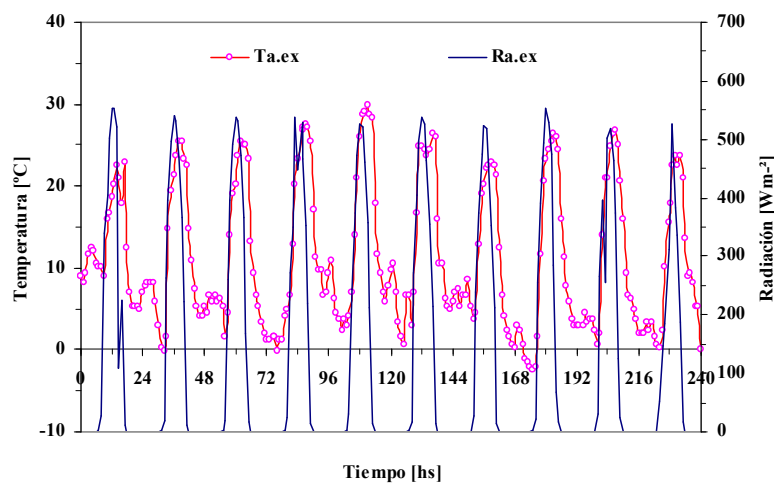
Fig. 4. Temperatura y radiación exterior para el primer periodo.
