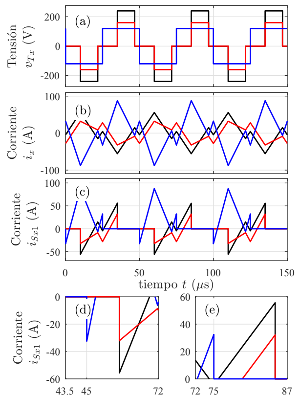
Figura 13: Resultados de simulación de caso 5, v_{T1} (negro), v'_{T2} (rojo) y v'_{T3} (azul) (a), i_1 (negro), i'_2 (rojo) y i'_3 (azul) (b), i_{S11} (negro), i_{S21} (rojo) e i_{S31} (azul) (c). En (d) se muestra un detalle de i_{Sx1} en el instante del encendido y en (e) en el instante del apagado.
