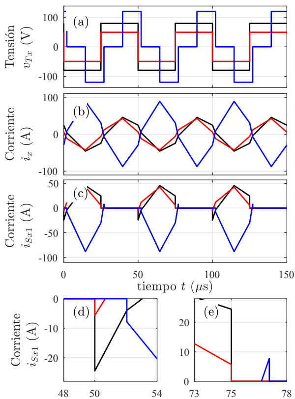
Figura 11: Resultados de simulación del caso 4, v_{T1} (negro), v'_{T2} (rojo) y v'_{T3} (azul) (a), i_1 (negro), i'_2 (rojo) y i'_3 (azul) (b), i_{S11} (negro), i_{S21} (rojo) e i_{S31} (azul) (c). En (d) se muestra un detalle de i_{Sx1} en el instante del encendido y en (e) en el instante del apagado.
