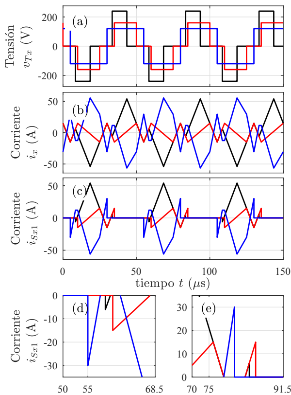
Figura 15: Resultados de simulación del caso 6, v_{T1} (negro), v'_{T2} (rojo) y v'_{T3} (azul) (a), i_1 (negro), i'_2 (rojo) y i'_3 (azul) (b), i_{S11} (negro), i_{S21} (rojo) e i_{S31} (azul) (c). En (d) se muestra un detalle de i_{Sx1} en el instante del encendido y en (e) en el instante del apagado.
