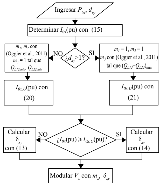
Figura 4: Diagrama de flujo del algoritmo de modulación propuesto.
