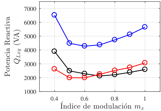
Figura 12: Potencia reactiva en cada inductancia del circuito equivalente en \Delta Q_{L13} (negro), Q_{L23} (rojo) y Q_{L13} + Q_{L23} (azul) en función del índice de modulación m_x para el caso 4.
