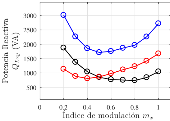
Figura 10: Potencia reactiva en cada inductancia del circuito equivalente en \Delta Q_{L13} (negro), Q_{L23} (rojo) y Q_{L13} + Q_{L23} (azul) en función del índice de modulación m_x para el caso 3.
