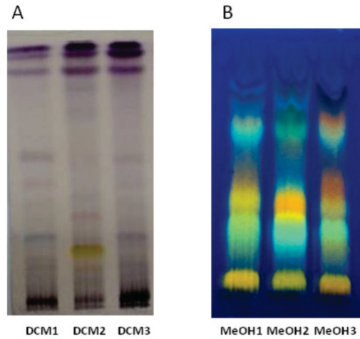
Fig. 2: Perfil cromatográfico por TLC de los extractos diclorometánicos DCM1, DCM2 y DCM3 y metanólicos MeOH1, MeOH2 y MeOH3. A: Extractos diclorometánicos FE: Silicagel 60 F254 FM: hexano:acetato de etilo (5:5). Revelado: anisaldehído sulfúrico (ANIS). B: Extractos metanólicos FE: Celulosa FM: ácido acético 15%. Revelado: reactivo 2-aminoetildifenilbórico (NPR).
