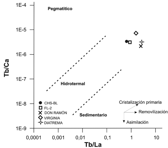
Figura 5: Fluoritas estudiadas representadas en un diagrama de variación Tb/Ca vs. Tb/La (Möller et al. 1976). Las tendencias de procesos pertenecen a O'Connor et al. (1993).
