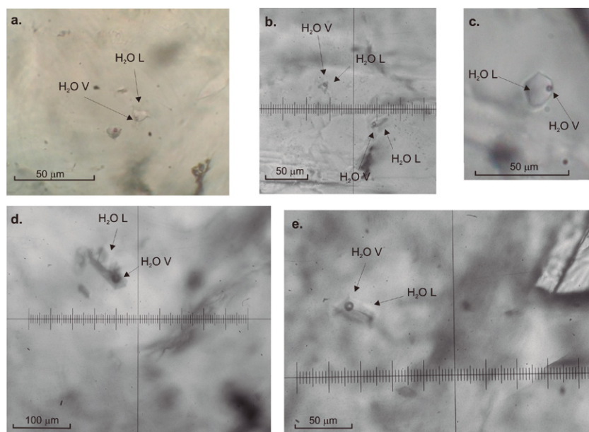
Figura 6: Inclusiones fluidas en fluorita utilizadas en las mediciones microtermométricas. a) Población de inclusiones fluidas primarias con fase líquida dominante en fluorita celeste de brecha Diatrema, yacimiento Chus-Chus; b) Conjunto de inclusiones fluidas primarias con fase líquida dominante en fluorita blanca de brecha Virginia, yacimiento Chus-Chus; c) Inclusión fluida en fluorita blanca de veta Don Ramón; d) Grandes cristales negativos concatenados con morfología de dodecaedros rómbicos de comportamiento metaestable, en fluorita violácea de la veta Ramón Arias, pertenencia Brackebusch, prospectos Pircas Coloradas; e) Inclusión fluida primaria con fase líquida dominante de fluorita de la pertenencia Bodenbender, prospectos Pircas Coloradas.
