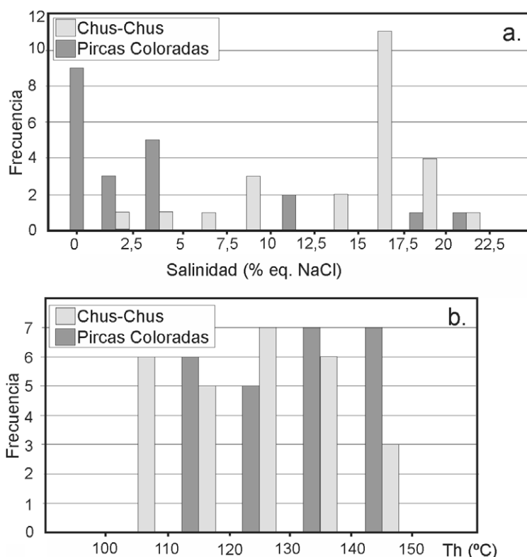
Figura 7: a) Histograma de frecuencia de salinidades (% eq. en peso de NaCl); b) Histograma de frecuencia de temperaturas de homogeneización ( T_h en °C).
