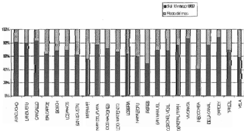
Figura 3. Distribución espacial de precipitaciones en el sudeste bonaerense en marzo de 1999 (% de la precipitación mensual total)
