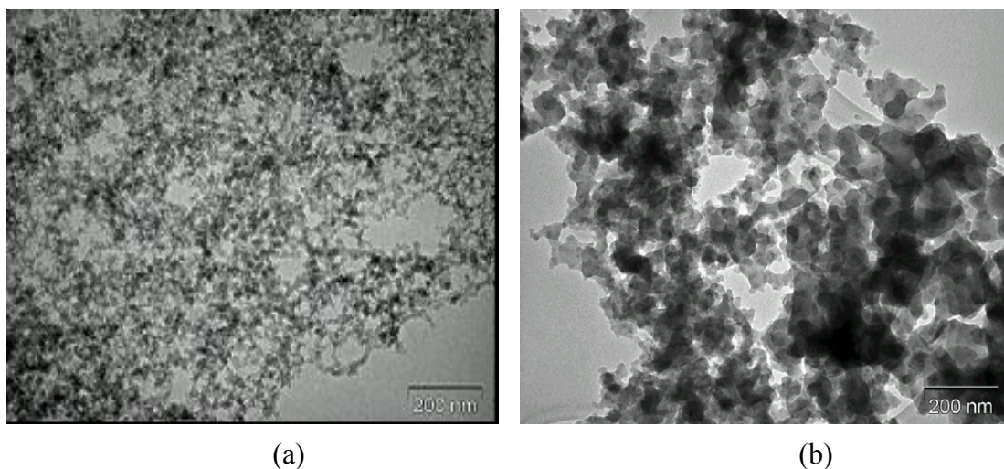
Figura 5. Micrografías TEM para la sílice: (a) sin modificar y (b) modificada con 3-aminopropiltriatoxisilano.
