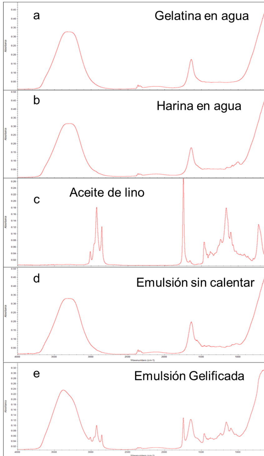
Figura 3: Espectros ATR-FTIR en los 2960\text{-}2830\text{ cm}^{-1} , correspondiente a la región de aceite de lino puro (c) y emulsión gelificada de aceite de oliva en agua (e), adicionados con harina de garbanzo.
