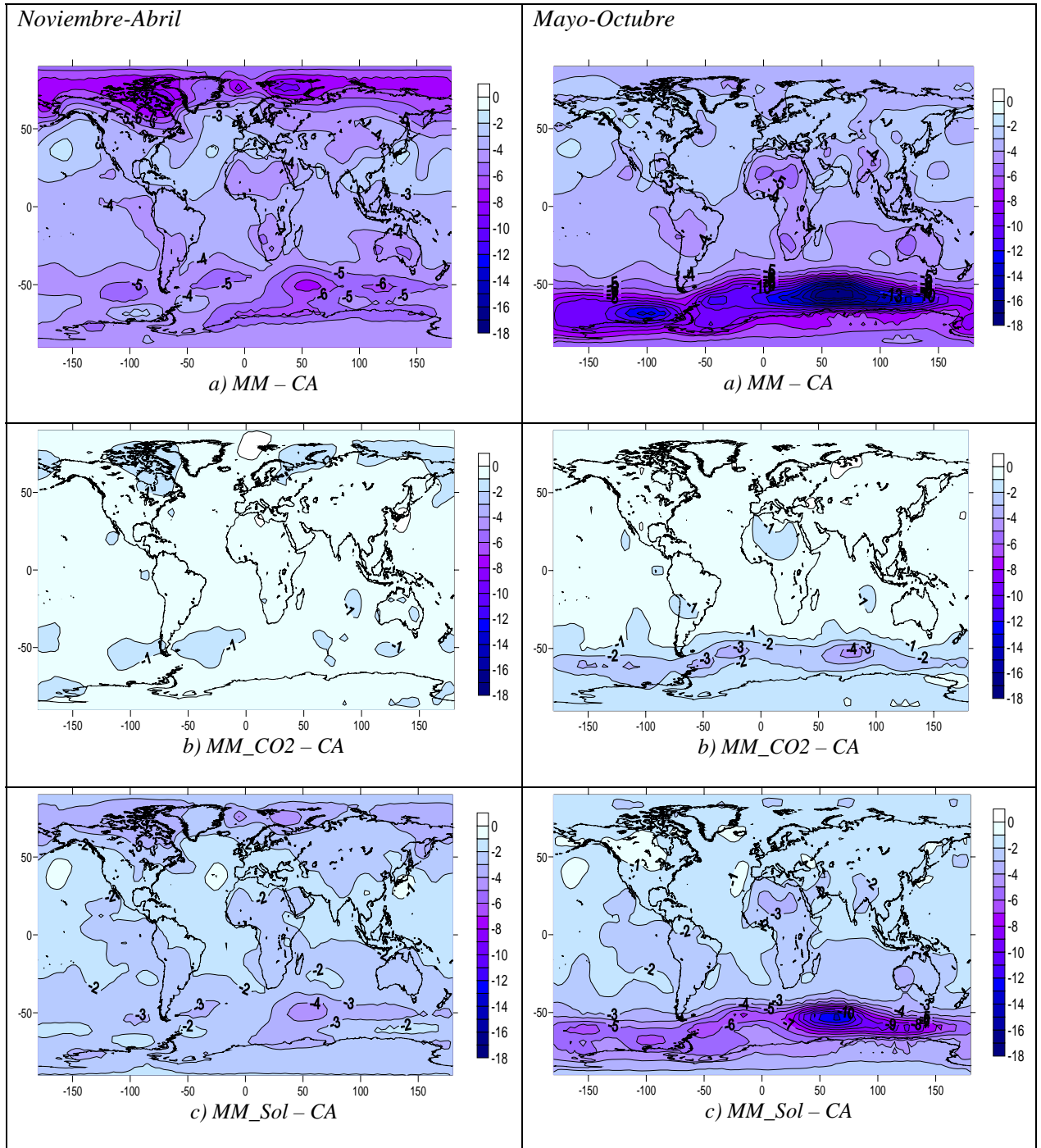
Figura 5. Anomalías de temperatura ( T^{\circ}\text{C} ) entre: a) MM y segunda mitad del siglo veinte (CA); b) irradiancia del MM, gases del MM y CO2 actual (MM_CO2) versus CA; c) concentración de gases del MM con irradiancia actual (MM_Sol) y CA (Ver Tabla 1). Semestre Noviembre-Abril (cálido para HS) en el panel izquierdo y Mayo-Octubre (frío para HS) en el panel derecho.
