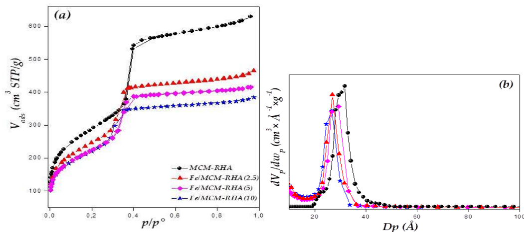
Figura 1. Isothermas de adsorción-desorción de N 2 a 77 K de los materiales bajo estudio.
