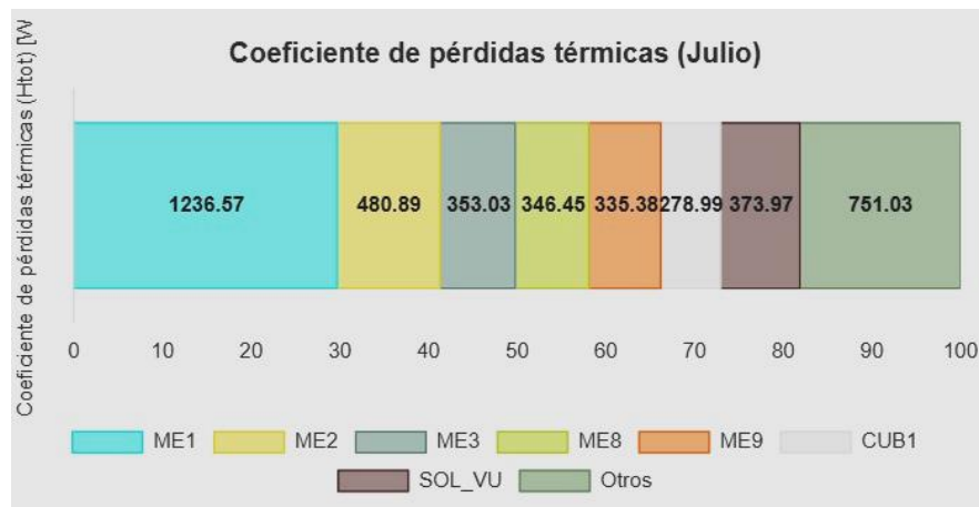
Fig. 9. Vivienda Universal –VU– DPVyU. Pérdidas Térmicas del Muro Exterior 1 –ME1– expresadas en KWh para el mes de Julio. Fuente: Aplicativo de etiquetado de Viviendas.
