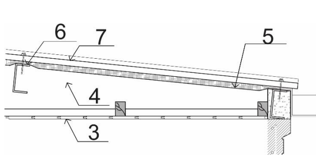
Fig. 6. Cubierta: 3. Machimbre de madera de Pino (1,5 cm). 4. Cámara de aire horizontal (Prom. 10,0 cm). 5. Barrera de Vapor (200 micrones). 6. Feltro de lana de vidrio (5,0 cm). 7. Chapa Galvanizada (Trapezoidal / Ondulada) (<0,1cm). Fuente: Elaboración Propia
