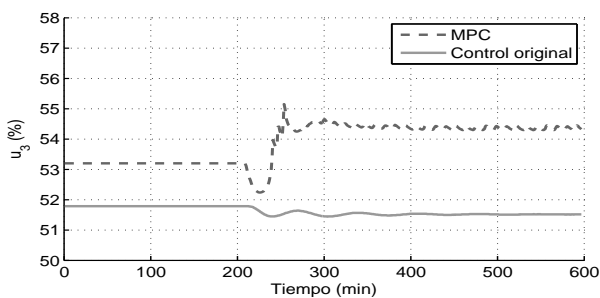
(c) Porcentaje de apertura válvula agua
