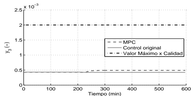
(c) Contenido de metanol en el biodiésel
