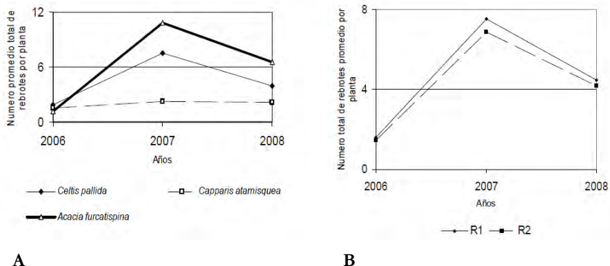
Figura 5 Efecto de rolados de baja (R1) y elevada (R2) intensidad, en especies arbustivas del Chaco de Argentina. A. Número promedio de rebrote por planta en Celtis pallida , Capparis atamisquea y Acacia gilliesii (Ex A. furcatispina ). B. Número promedio de rebrotes por planta con R1 y R2. Tomado de Kunst et al. (2009).
