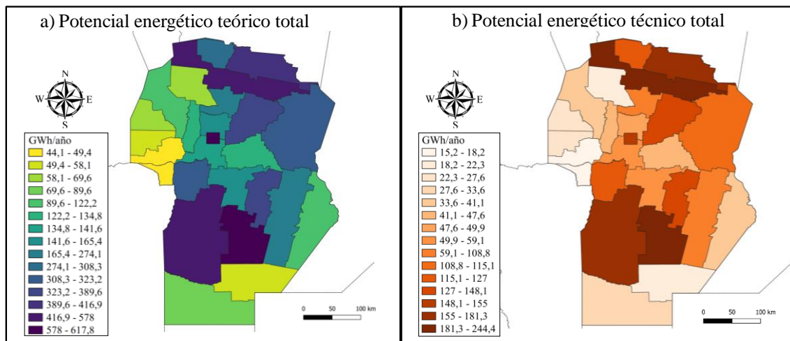
Figura 2 - Potencial energético a) teórico y b) técnico total, de acuerdo a la ecuación (4a y 4b).
