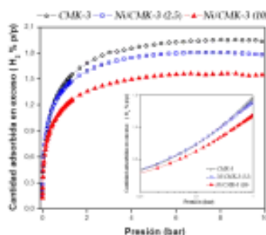
Figura 4. Isothermas de adsorción de H_2 a 77 K y 10 bar. Inset: isothermas de H_2 a 77 K y presiones menores a 1 bar en escala logarítmica.
