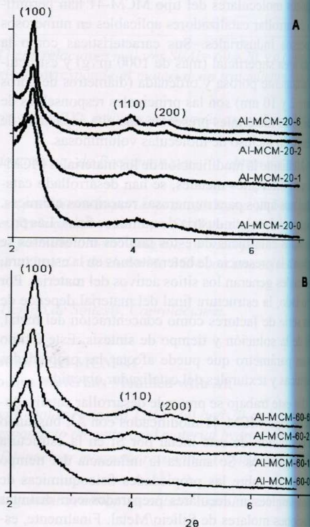
Figura 1: Patrones de DRX de: (A) Al-MCM-41, Si/Al=20 y (B) Al-MCM-41, Si/Al= 60
