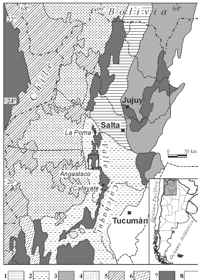
Figura 1: El Valle Calchaquí y las provincias geológicas del norte argentino (adaptado de Salfity y Marquillas 1994). El recuadro indica la ubicación de la figura 2. 1) Cordillera Oriental, 2) Sierras Pampeanas Septentrionales, 3) Sierras Subandinas, 4) Puna, 5) Arco volcánico de la Cordillera Principal, 6) Sistema de Famatina, 7) Depresiones cuaternarias y 8) Llanura Chaqueña.
