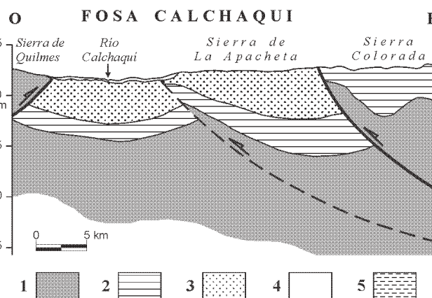
Figura 2: Arriba: Mapa geológico simplificado de la porción central del Valle Calchaquí (adaptado de Salfity y Monaldi, 1998). Ubicación: véase Figura 1. A-B Corte estructural. 1) Basamento metamórfico-ígneo precámbrico-paleozoico, 2) Grupo Salta (Cretácico-Paleógeno), 3) Grupo Payogastilla (Neógeno) (se indica las curvas de nivel más elevadas de la sierra de La Apacheta y la línea de su cumbre), 4) Cuaternario, 5) Supuesta dispersión del lago cuaternario, según la curva de nivel actual, aproximada, de 1.900 m sobre el nivel del mar. Se indica también la curva de nivel de 2.000 metros s.n.m. Abajo: Corte estructural esquemático A-B, no balanceado, a lo largo del paralelo 25°36' LS. Las referencias son idénticas a las del mapa geológico.
