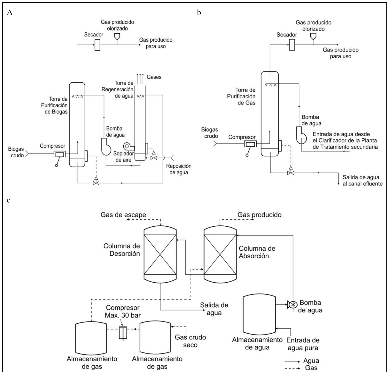
Fig. 1. Esquemas de purificación de biogás por absorción acuosa
