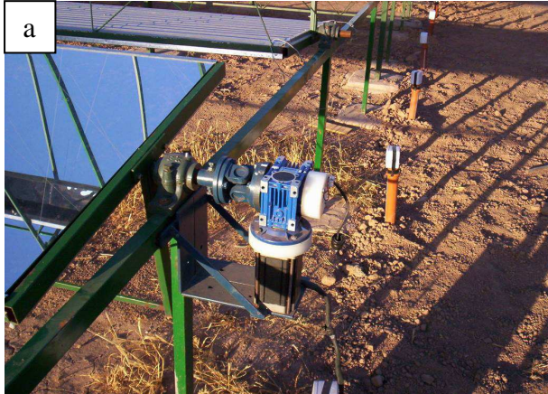
Fig. 12a.-El motor paso a paso que proporciona el giro a las filas de espejos y la caja azul de demultiplicación Fig. 12b.-Gabinete con los elementos electrónicos utilizados para comandar los motores.
