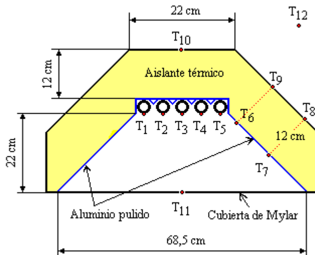
Figura 5.- Esquema de la sección transversal de un absorbedor mostrando los caños y la aislación.
