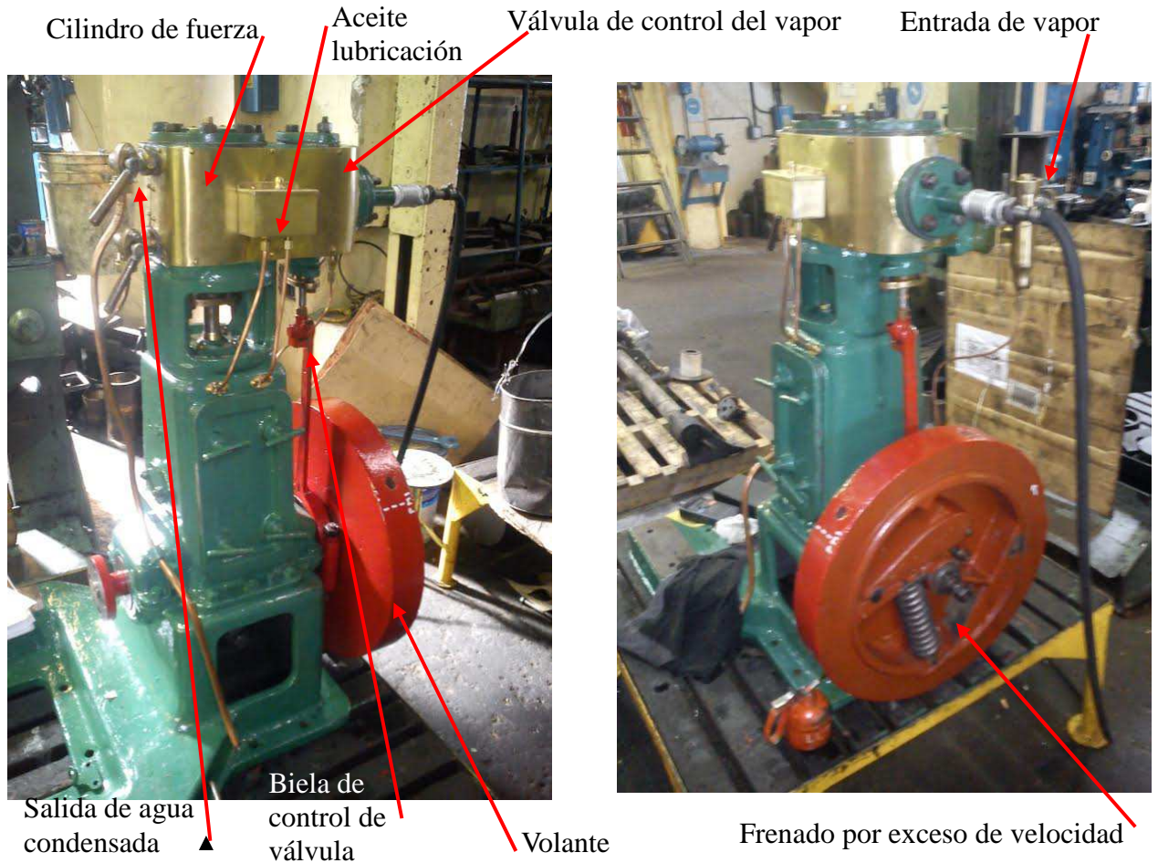
Figuras 14 a y 14 b.- Dos vistas del motor de vapor de 17 HP a 300 rpm.
