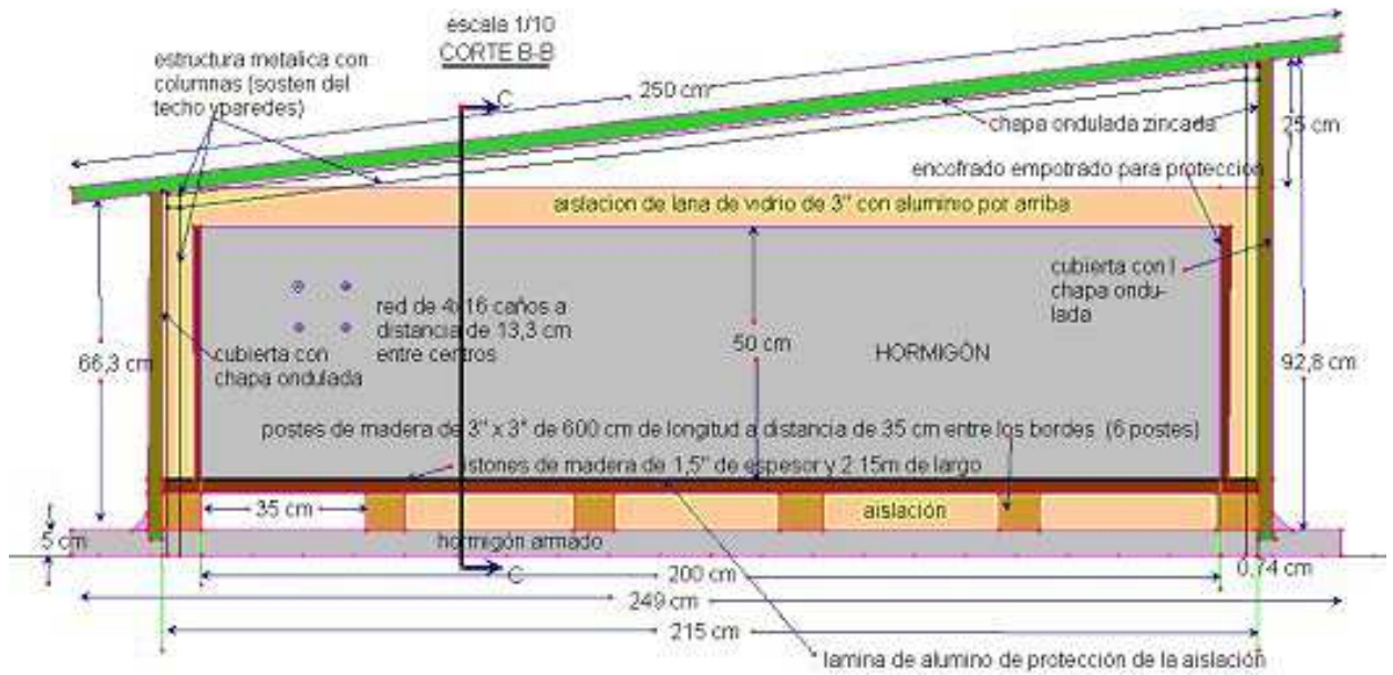
Figura 8. Corte transversal del acumulador mostrando los distintos materiales que lo forman.
