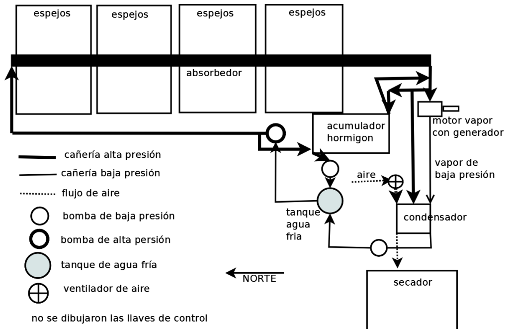
Figura 1.- Esquema de la planta del generador solar térmico de tipo fresnel y sus diferentes partes. No se indican las válvulas.
