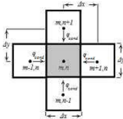
Figura 6: Transferencia conductiva en un volumen de control
