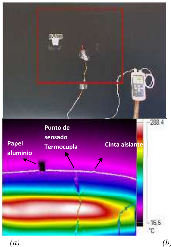
Figura 7. (a) Imagen visible. (b) termograma de la cara posterior de la pantalla.
