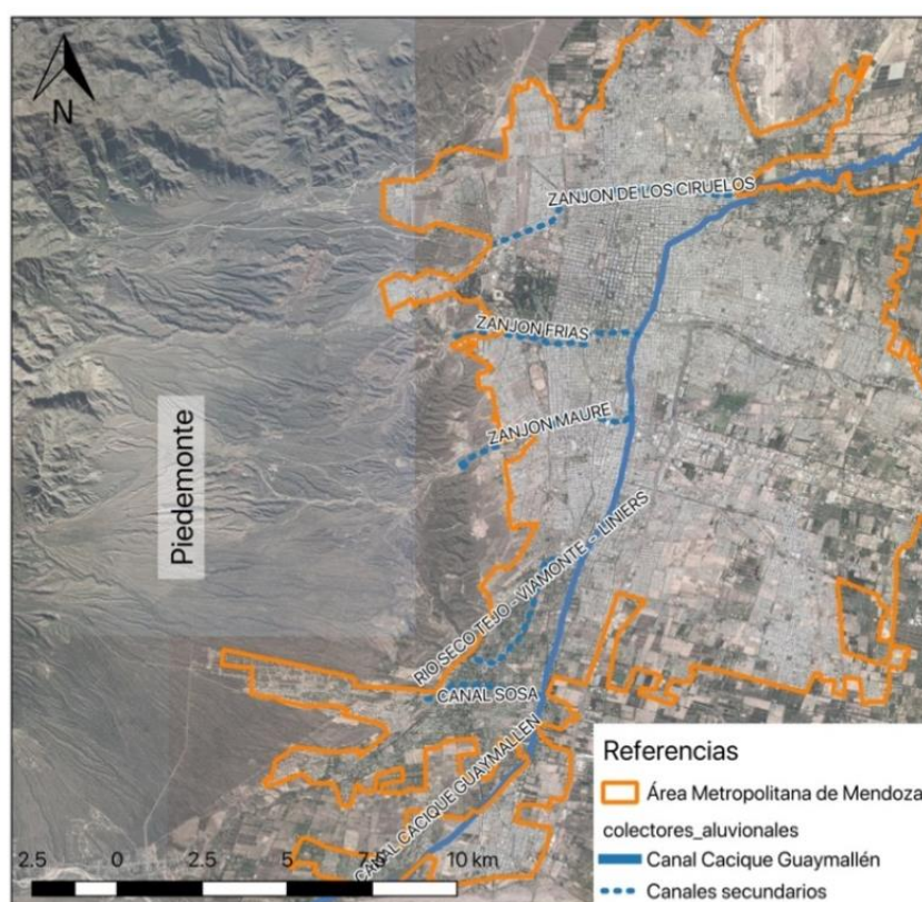
Figura 4.- Sistema de corrección aluvional del Área Metropolitana de Mendoza. Fuente: Elaboración propia a partir de información suministrada por el Departamento General de Irrigación.
