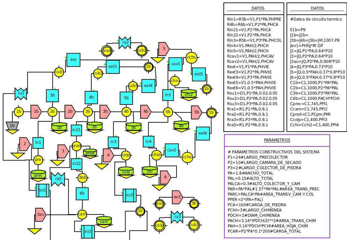
Figura 4: Circuito térmico para el secador propuesto. Se indican los cuadros entrada de datos y parámetros constructivos.
