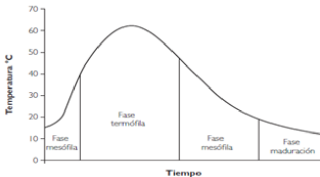
Figura 20: fases del proceso de compostaje en relación a los cambios de temperatura. Se puede observar que en la fase termófila las temperaturas superan los 60°C pudiendo alcanzar los 70°C. Fuente: Mazzarino et.al. , 2012.
