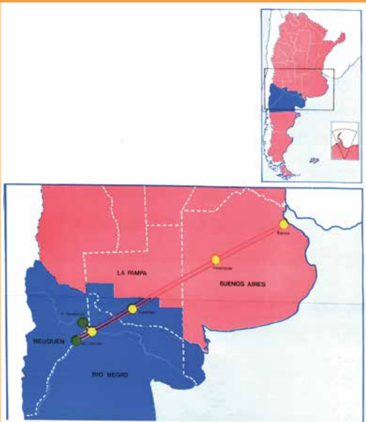
Figura 3: Esquema de las líneas de transmisión energética.
