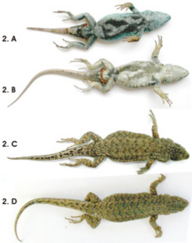
Figura 2. Vistas ventrales de L. coeruleus macho (2.A) y L. neuquensis macho (2.B). Vistas dorsales de L. coeruleus hembra (2.C) y L. neuquensis hembra (2.D). Fotos: J.A. Scolaro, febrero 2006 Figure 2. Ventral views of L. coeruleus male (2.A) and L. neuquensis male (2.B). Dorsal views of L. coeruleus female (2.C) and L. neuquensis female (2.D). Photos: J.A. Scolaro, february 2006
