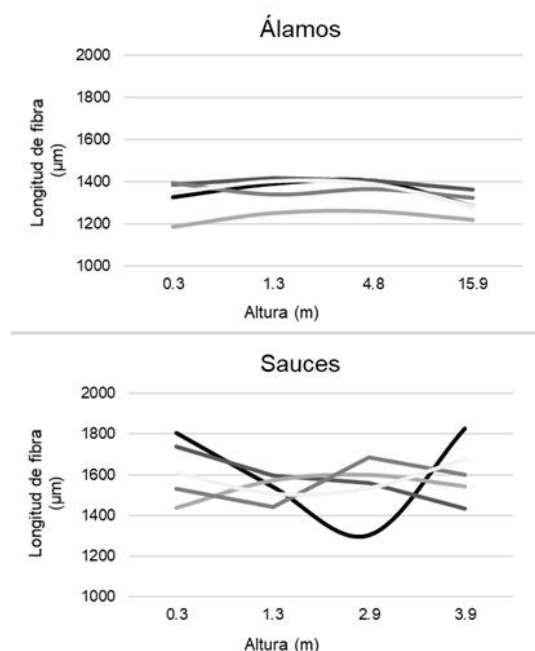
Figura 2. Variación de la longitud de fibra ( \mu\text{m} ) de álamos y sauces en función de la altura.
