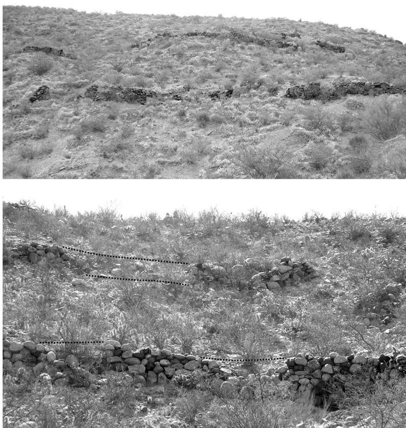
Figura 2. Ejemplos de murallas defensivas. Arriba: ladera occidental del Cerro Colorado (La Ciénaga de Abajo). Abajo: ladera occidental del Pueblo Viejo de El Eje; las líneas punteadas indican los sectores derrumbados
