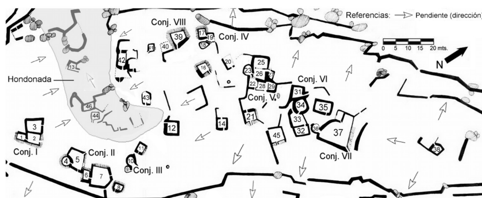
Figura 6. Detalle de los conjuntos de estructuras intrasitio de Loma de los Antiguos de Asampay.
