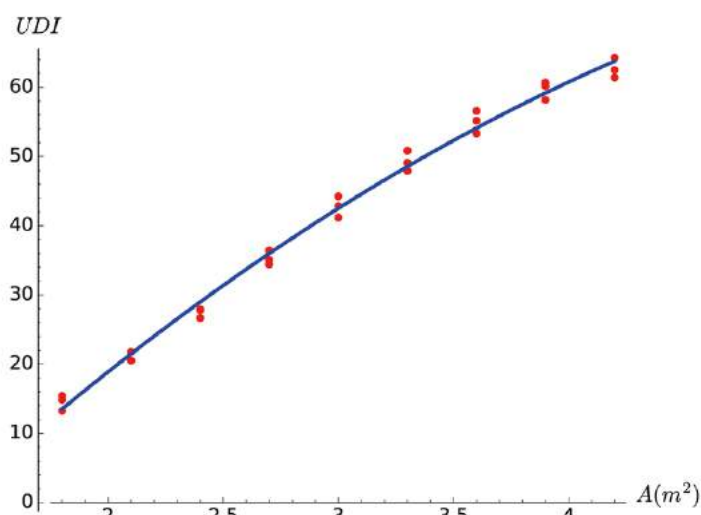
Figura 4. Datos y ajuste cuadrático para la orientación sur. Fuente: Elaboración del autor.
