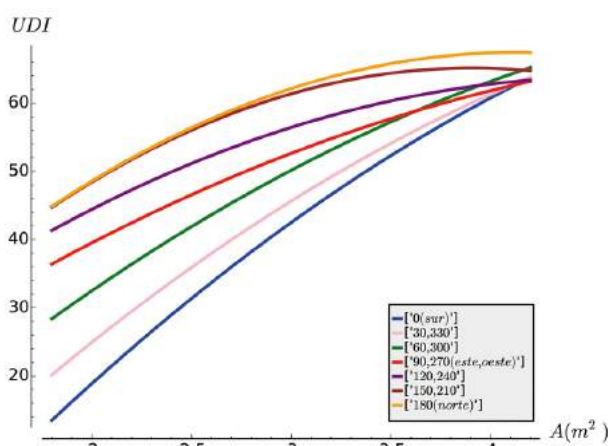
Figura 5. Curvas de ajustes obtenidos de UDI_{100-2000lx} de acuerdo al área vidriada y la orientación. Fuente: Elaboración del autor.
