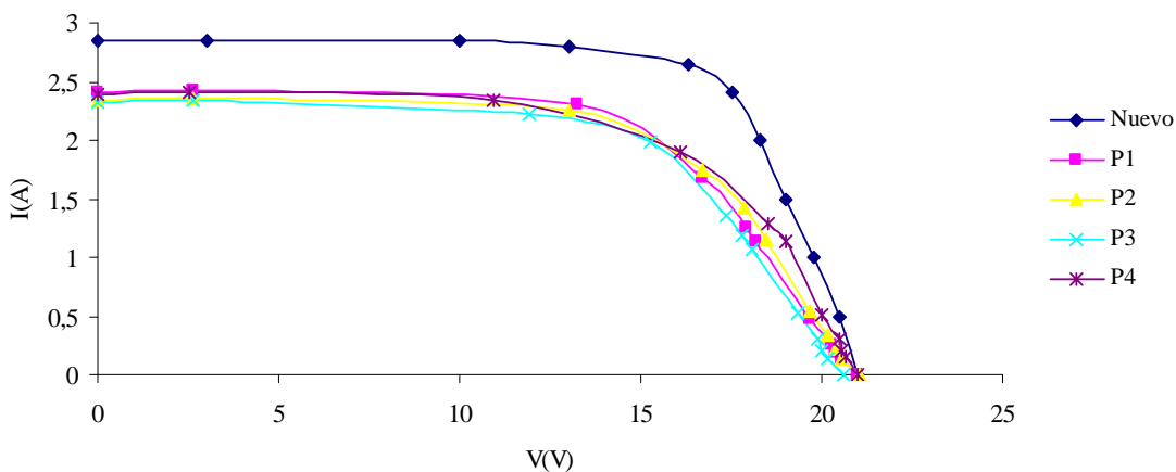
Figura 2: Curvas características I-V del conjunto de módulos Solarwatt.
