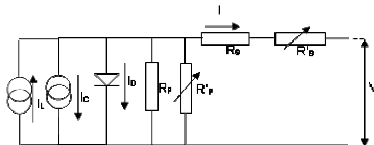
Figura 10. Modelo de circuito equivalente de un módulo degradado
