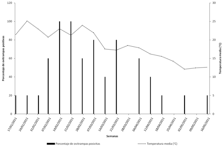
Fig. 2. Porcentaje semanal de ovitrampas conteniendo huevos de Aedes aegypti y temperatura media semanal, correspondientes al período comprendido entre el 17 de enero y el 16 de mayo de 2011.
