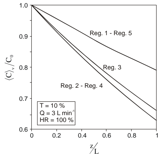
Figura 4. Concentración adimensional promedio, pesada en velocidades, para distintas alturas. Irradiación bilateral.
