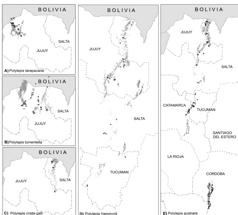
Figura 1. Distribuci n potencial de las especies de Polylepis descriptas en Argentina (en gris dentro de Argentina). Los  rculos negros representan los puntos de presencia conocidos con los cuales se confeccionaron los modelos de distribuci n potencial.
