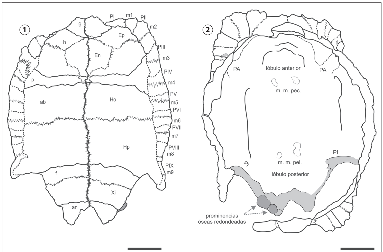
Figura 4. Ch. lutzae sp. nov. (CTES-PZ 7391 holotipo). 1 , vista ventral y esquema del plastrón; líneas en zigzag indican suturas (entre placas), líneas rectas indican surcos (entre escudos). Escala= 150 mm. 2 , vista visceral y esquema del plastrón. La flecha gris indica el engrosamiento visceral de la región lateral izquierda del xifoplastrón. Escala= 150 mm. Gris claro indica engrosamiento óseo, y gris oscuro indica prominencias óseas redondeadas. Escudos: ab , abdominal; an , anal; f , femoral; g , gular; h , humeral; m , marginal; p , pectoral. Placas: En , entoplastrón; Ep , epiplastrón; Ho , hio-plastrón; Hp , hipoplastrón; P , periférica; PA , pilares axilares; PI , pilares inguinales; PV , pigal; Xi , xifoplastrón. Marcas de musculatura en el plastrón: m.m.pec. , marcas de musculatura pectoral; m.m.pel. , marcas de musculatura pélvica.
