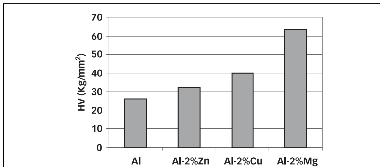
FIGURA 5: Valores de microdureza para una misma concentración de elemento aleante utilizando una carga de 100 g.
