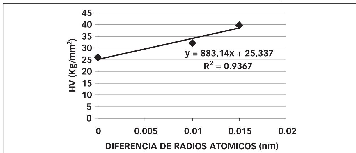
FIGURA 6: Valores de microdureza en función de la diferencia de radios atómicos utilizando una carga de 100 g.
