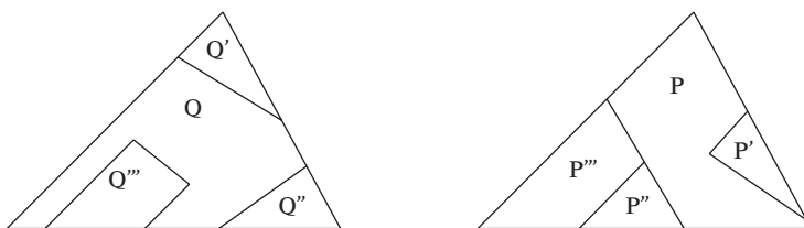
Fig. 3: Polígonos equicomplementarios.
