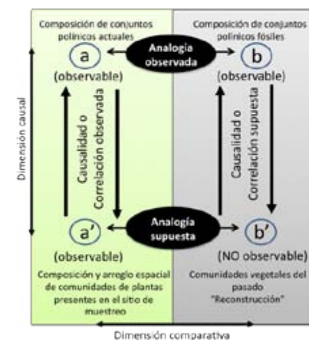
Figura 2. Diagrama esquemático de la lógica del razonamiento por analogía (modificado de Jackson y Williams, 2004).
