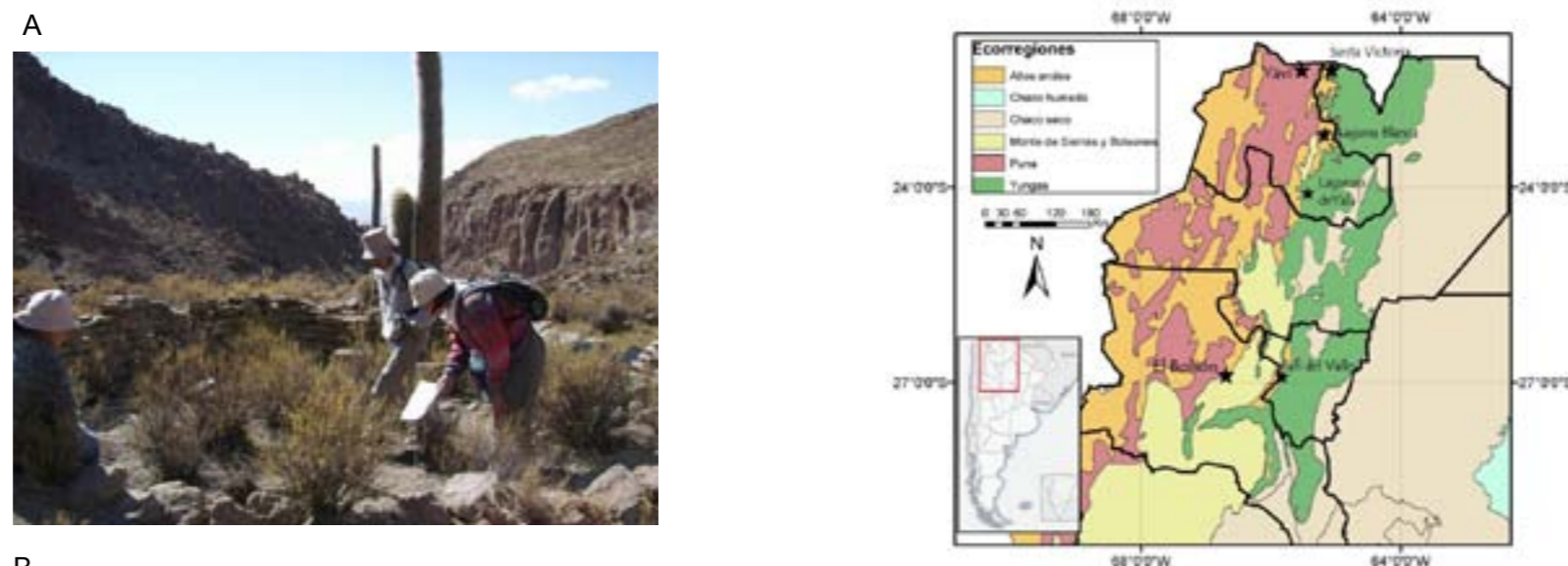
Figura 10. Mapa de ubicación de los sitios estudiados.
