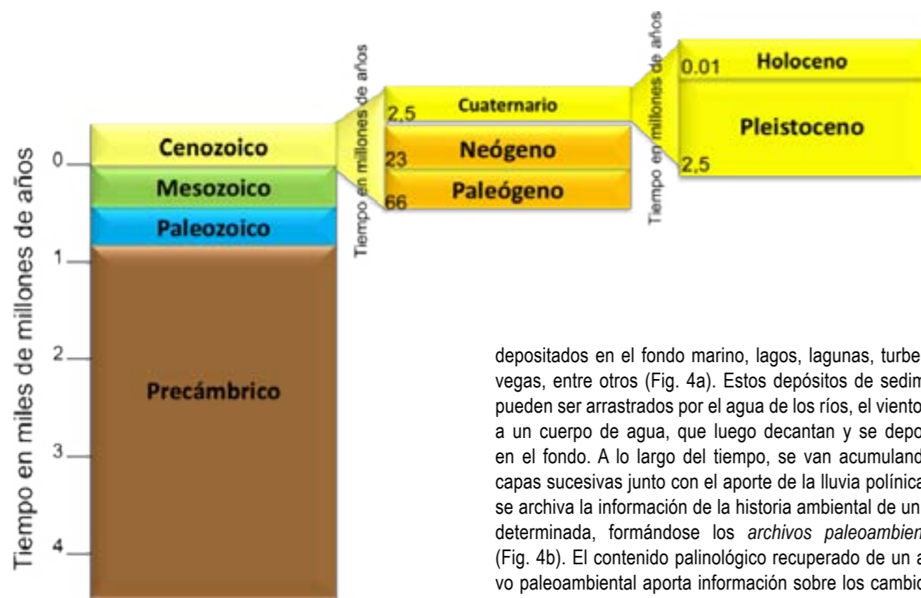
Figura 3. Escala general de tiempo geológico.
