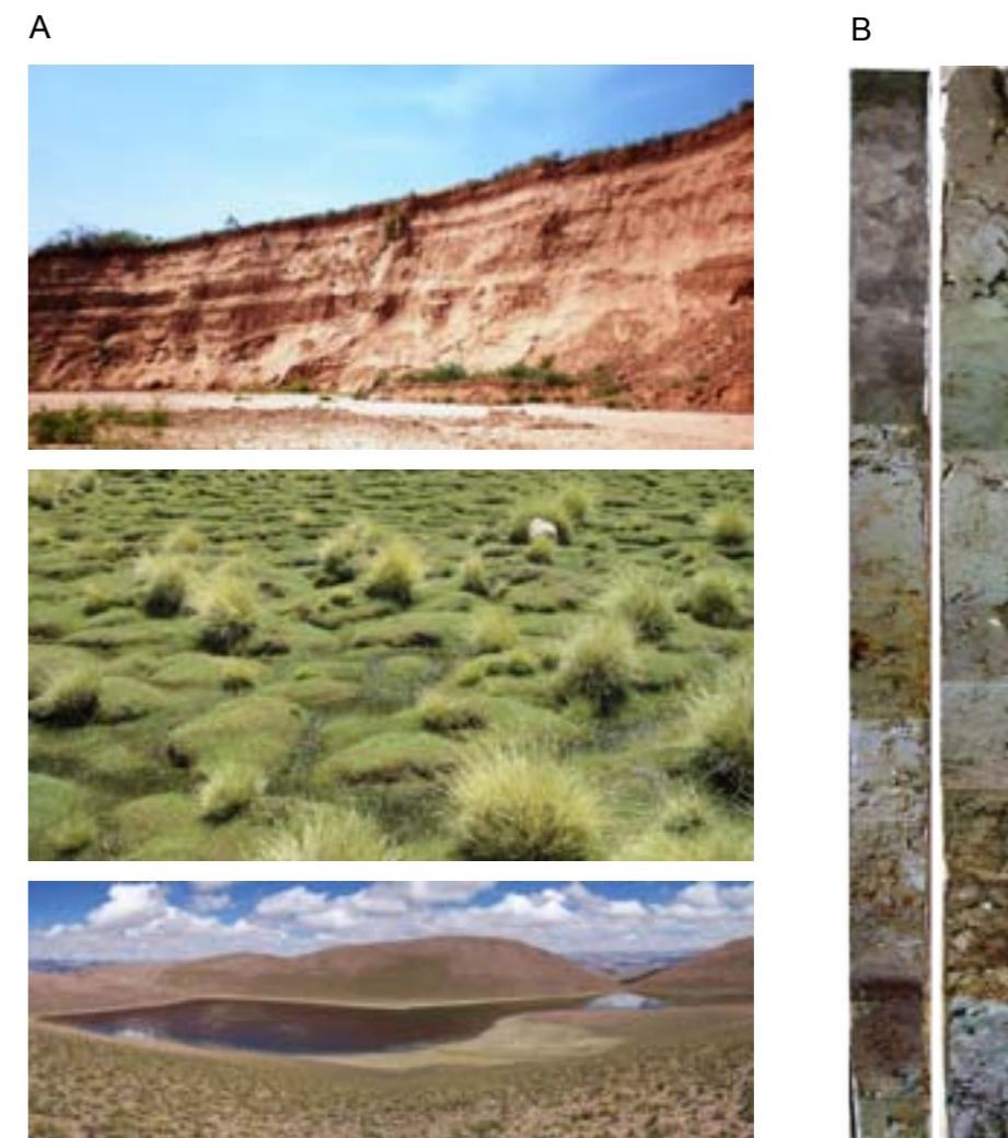
Figura 4. A) Ambientes sedimentarios. 1- Perfil aluvial. 2- Vega o turbera altoandina. 3- Laguna. B) Archivo paleoambiental, ejemplo de un testigo sedimentario "lacustre".
