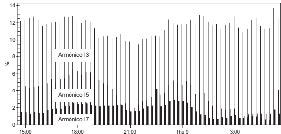
Fig. 16. Evolución de los componentes armónicos 3, 5 y 7 en la banda horaria 15:00 - 6:00 hs de la fase 1 Fuente: Autores.
