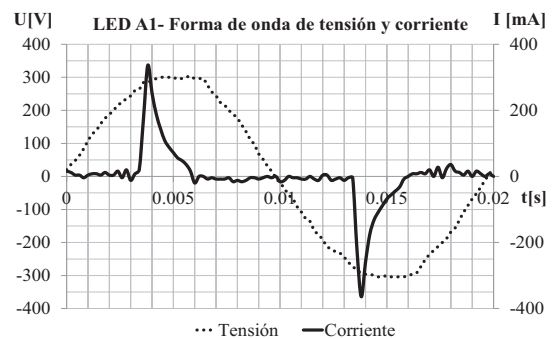
Fig. 2a. Forma de onda de tensión y corriente de una lámpara LED Fuente: Autores.
