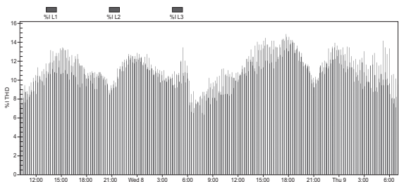
Fig. 17. Variación del THDI en las tres fases entre las 11:00 y 7:00 hs Fuente: Autores.
