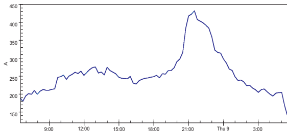
Fig. 15. Variación de la componente fundamental de corriente en la fase 1 a lo largo de un día Fuente: Autores.
