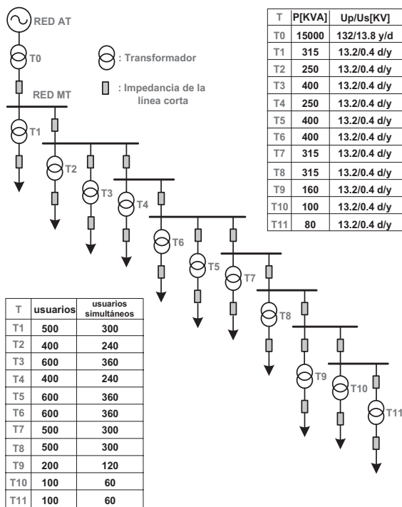
Fig. 11. Diagrama unifilar reducido de la red analizada Fuente: Autores.
