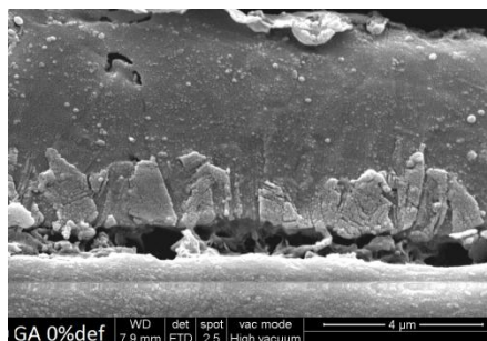
Figura 2. Metalografía de “galvanneal” comercial sin deformar.
