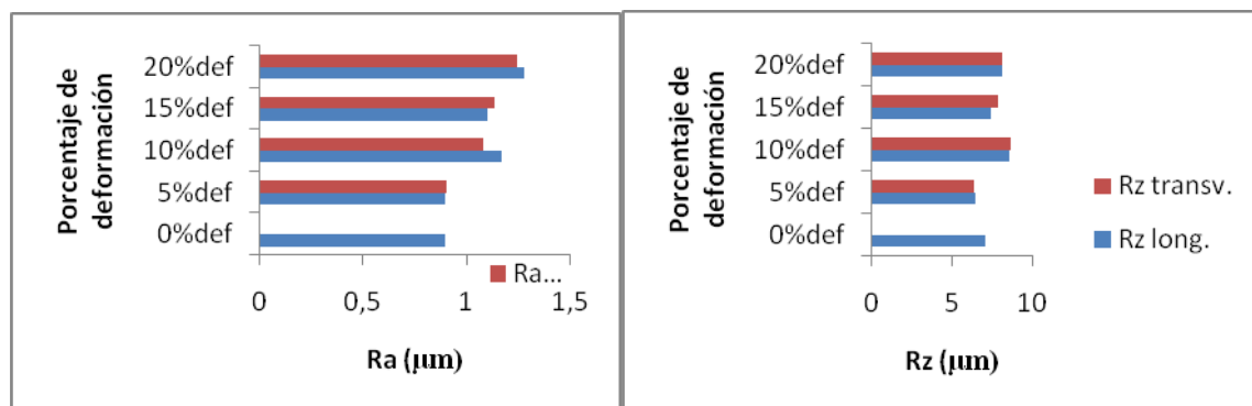
Figura 7. Comparación de valores de Ra, Rz
