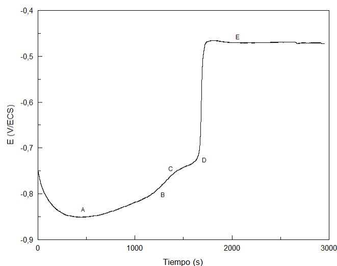
Figura3. Curva potencial (E) vs. tiempo obtenida del ensayo de stripping sobre “galvanneal” sin deformar.
