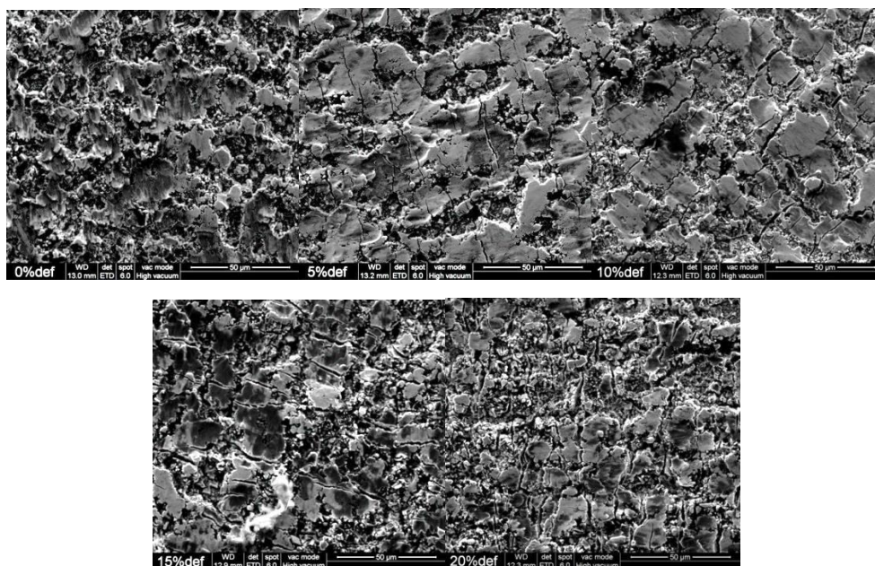
Figura 5. Fotografías de las superficies de “galvanneal” comercial con diferentes grados de deformación, obtenidas por microscopía electrónica.
