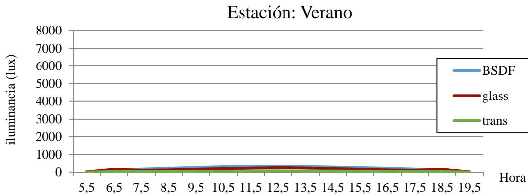
Figura 9: Gráfica de línea que muestra los valores de iluminancia en el nodo 5 para un día típico de verano.
