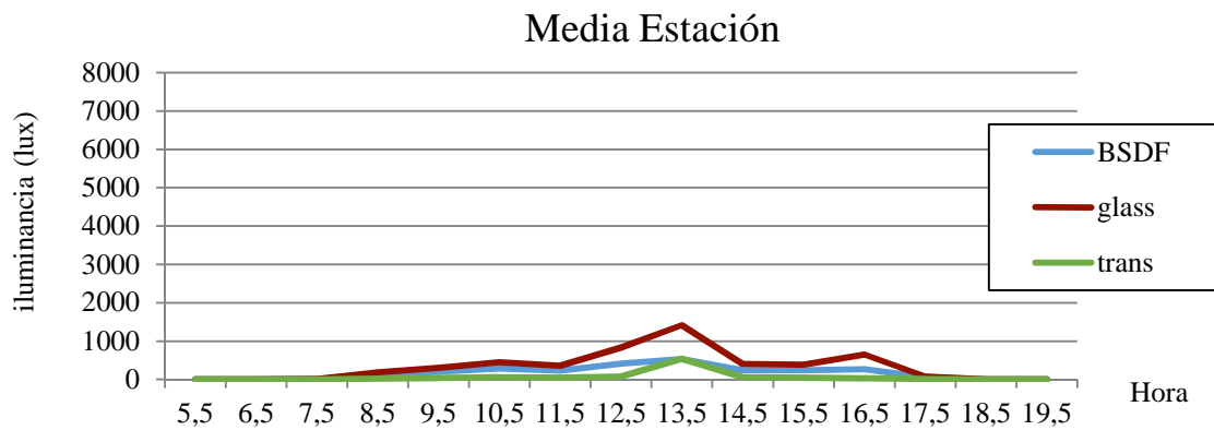
Figura 8: Gráfica de línea que muestra los valores de iluminancia en el nodo 5 para un día típico de media estación.
