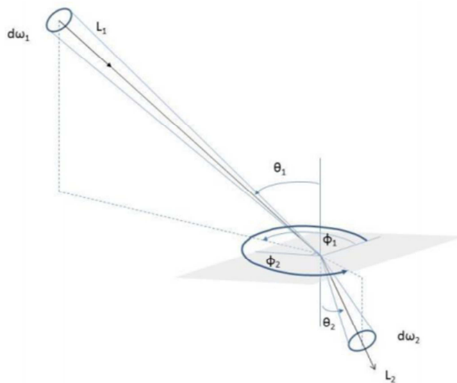
Figura 1: Gráfico de la geometría de la BSDF. (\theta_1, \phi_1) son las coordenadas polares del flujo luminoso incidente; (\theta_2, \phi_2) son las coordenadas polares del flujo luminoso transmitido; L_1(\theta_1, \phi_1) luminancia de un elemento producto del flujo luminoso incidente; L_2(\theta_2, \phi_2) luminancia de un elemento producto del flujo luminoso transmitido; d\omega_1 ángulo sólido subtendido por flujo de luz entrante; d\omega_2 ángulo sólido subtendido por flujo de luz incidente.
