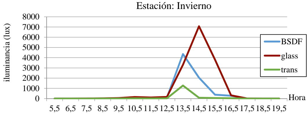
Figura 7: Gráfica de línea que muestra los valores de iluminancia en el nodo 5 para un día típico de invierno.
