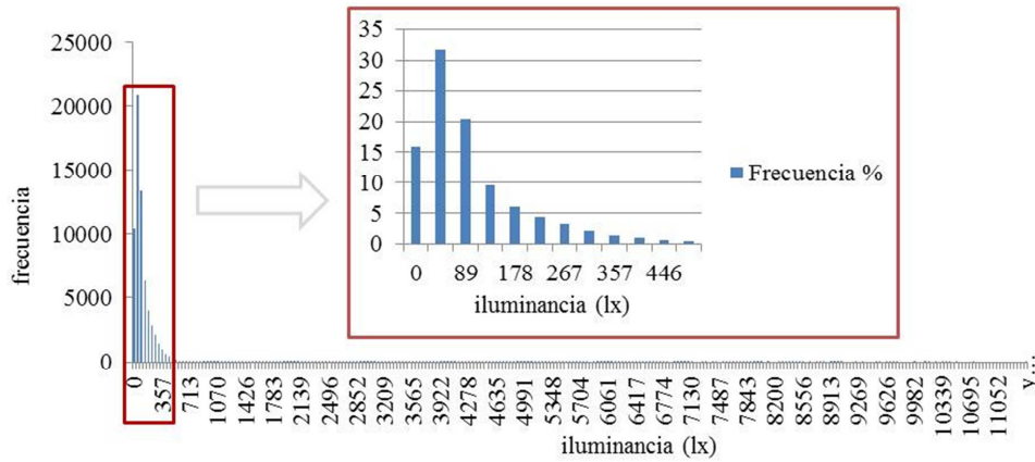
Figura 6: Histograma de los valores de iluminancia obtenidos mediante simulación de acuerdo a la condición BSDF.
