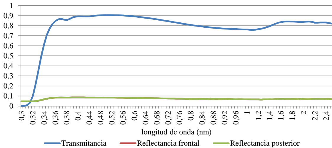
Figura 3: Gráfica que muestra la selectividad espectral del vidrio claro de 3mm seleccionado.
