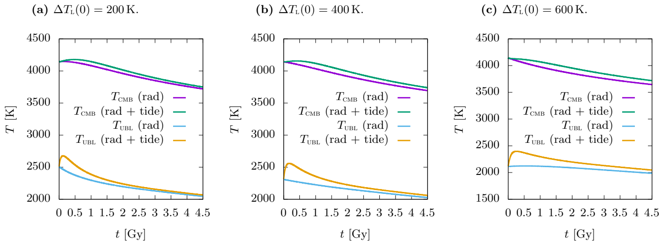
Figura 2: Gráficas de la evolución temporal de la temperatura en la CMB ( T_{\text{CMB}} ) y de la base de la capa límite inferior ( T_{\text{UBL}} ) teniendo en cuenta solamente el calor radiogénico (rad) y este junto al calor por mareas (rad + tide) para distintos valores iniciales del salto de temperatura entre la CMB y la parte superior de la capa límite inferior.
