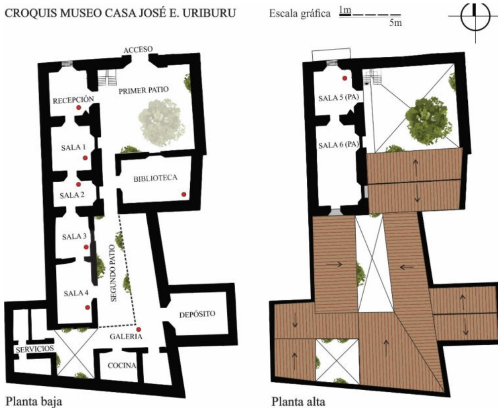
Figura 3: Croquis del Museo Planta Baja y Planta Alta. Los círculos rojos señalan la ubicación de los sensores de medición. Fuente: elaboración propia.
