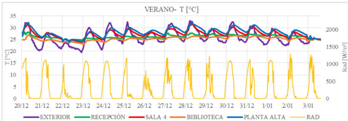
Figura 6: Grafico de Temperaturas monitoreadas durante periodo de verano (19/12/20 al 04/01/21). Fuente: elaboración propia.
