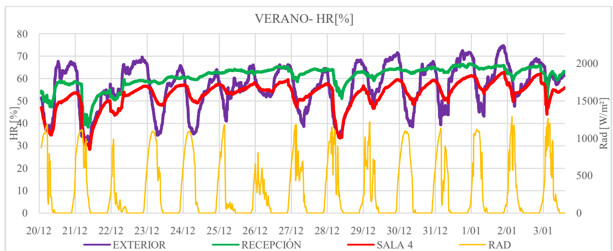
Figura 7: Grafico de contenido de humedad calculado para el periodo de verano (19/12/20 al 04/01/21). Fuente: elaboración propia.
