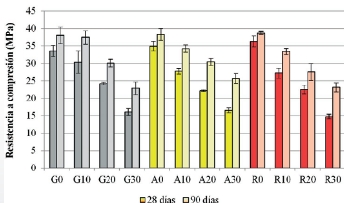
Figura 7 Resistencia a compresión a 28 y 90 días Fuente: Propia
