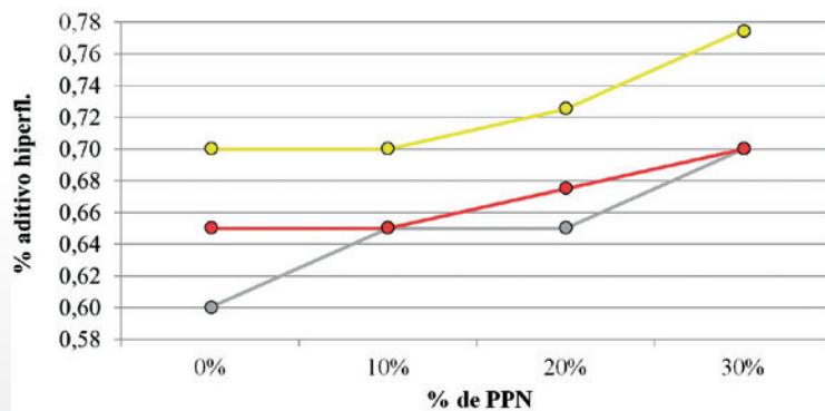
Figura 2 Dosis de aditivo Fonte: Propia
