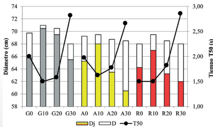
Figura 3 Slump-flow y J-Ring Fonte: Propia
